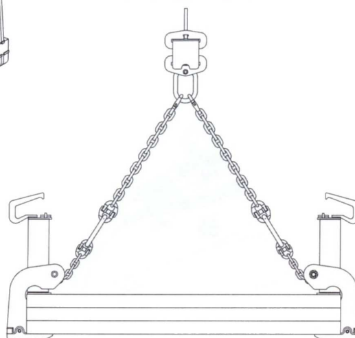
TLH/TLR/TLC
