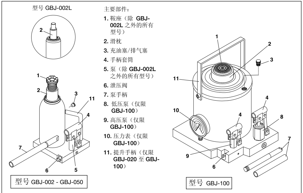
图 2 - 功能和组件
