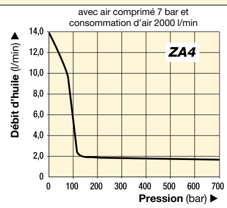
Série ZA4 avec réservoir 10 - 20 - 40 litres
