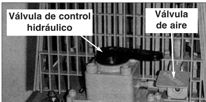
Figura 6 - Controles de la bomba
