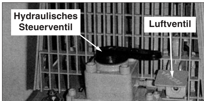
Abbildung 6 - Pumpensteuerungen
