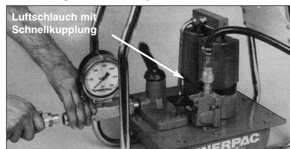
Abbildung 5 - EAM-Pumpe mit Lufteinlaßanschluß
