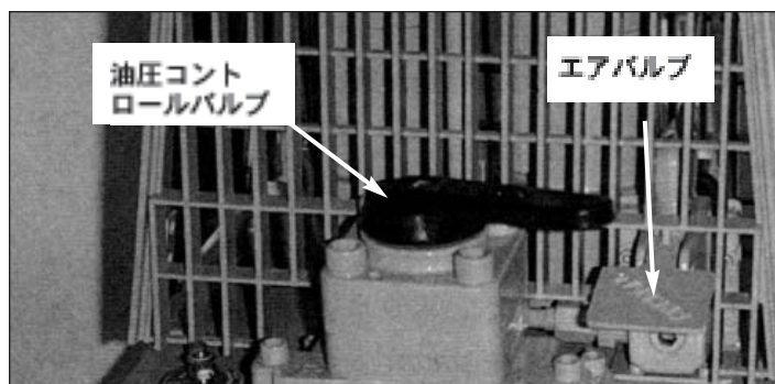
図6 - ポンプ制御装置
