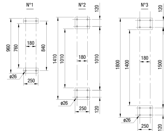
Détail des fixations / Fixation information / Details aus Befestigungen
